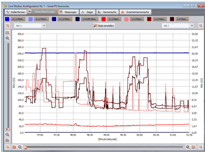
Abb. 47. Diagramm der Echtzeitwerte.
