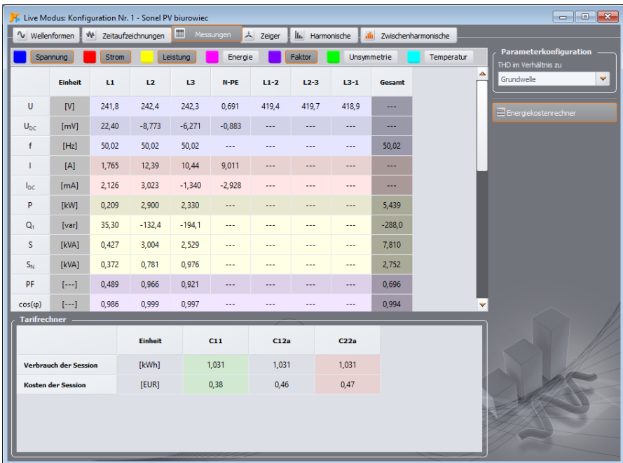
Abb. 48. Anzeige von Phasen- und Summenwerten.
