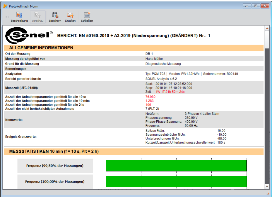
Abb. 65. Messbericht über die Übereinstimmung mit der Norm.
