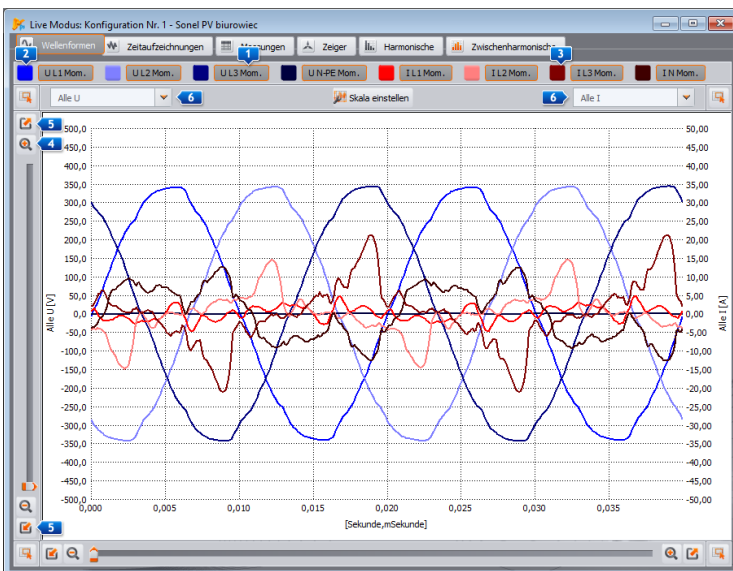
Abb. 45. Bildschirm im aktuellen Datenlesemodus - Wellenformen.
