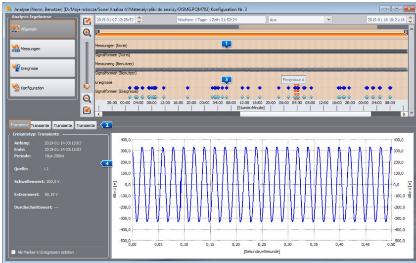
Abb. 57. Fenster ALLGEMEIN mit Oszillogramm-Vorschau.
