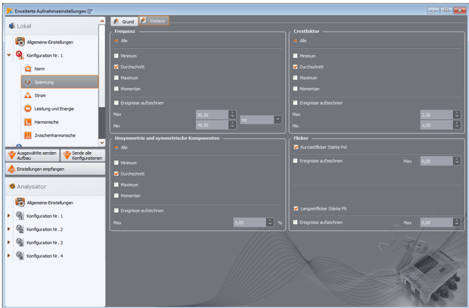
Abb. 24. Zusätzliche Einstellungen für Spannungsmessungen.
