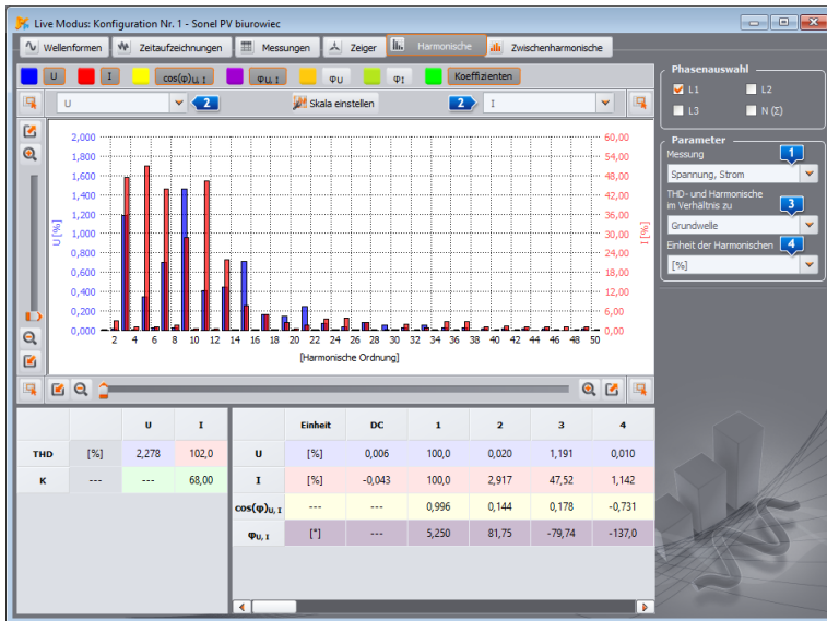
Abb. 50. Aktuelle Oberwellenwerte.
