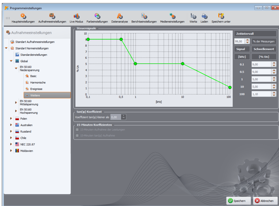
Abb. 81. Aufzeichnung nach EN 50160 – zusätzliche Einstellungen.
