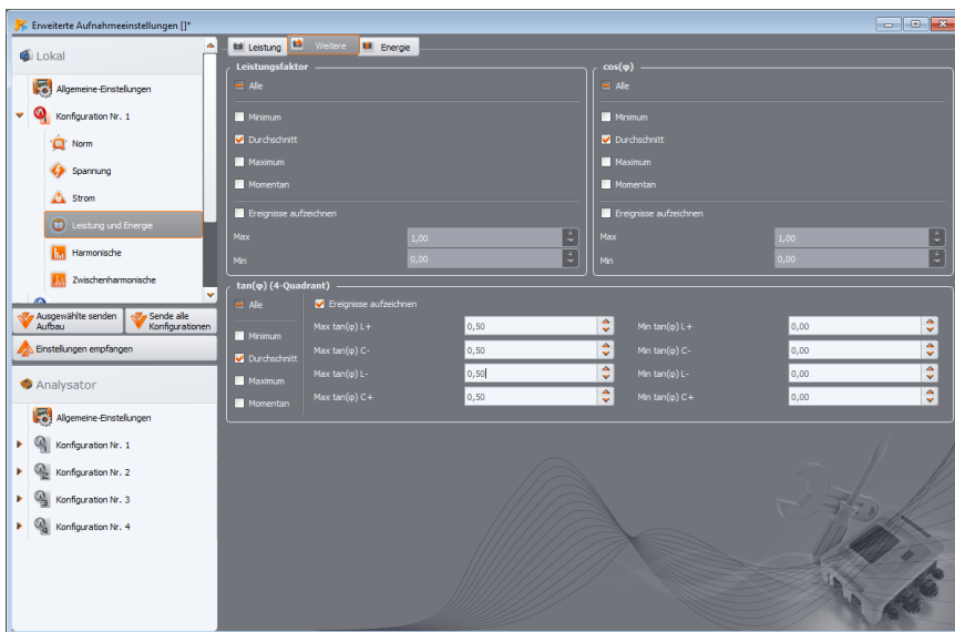
Abb. 27. Leistung und Energie: Registerkarte Weitere.
