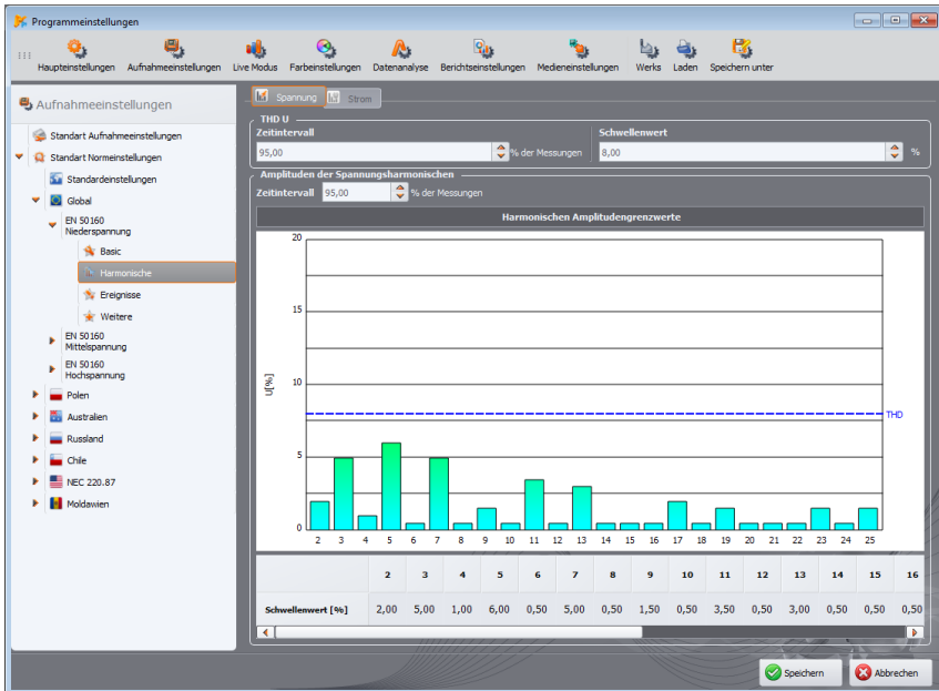
Abb. 79. Aufzeichnung nach der Verordnung - Einstellungen der Harmonischen.
