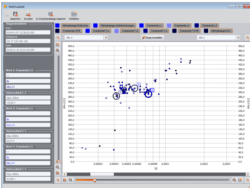
Abb. 70. Ereignisanalyse – Diagramm Wert/Laufzeit.
