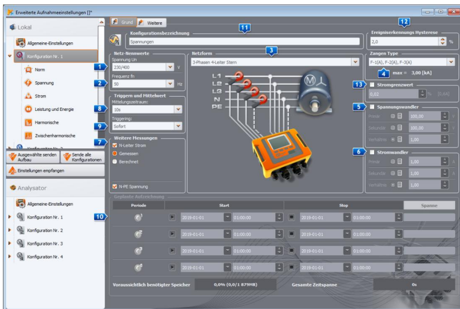
Abb. 20. Einstellungen für Netztyp, Netzleistungen und Wandler.
