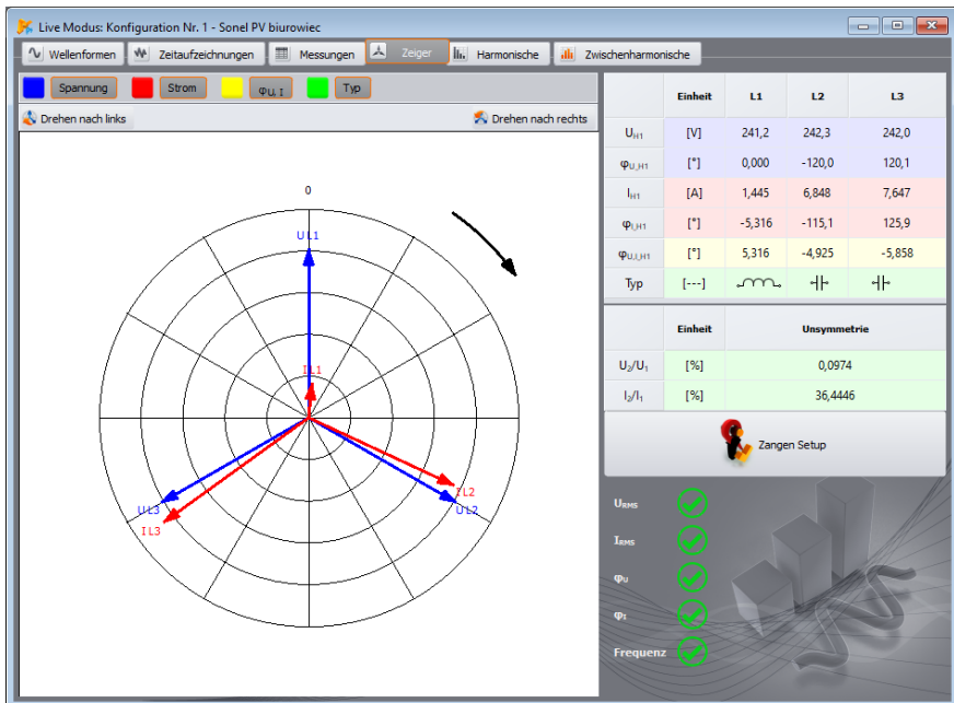
Abb. 49. Zeigerdiagramm für Sternschaltung.
