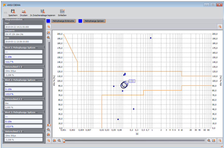
Abb. 71. Diagramm ANSI/CBEMA.
