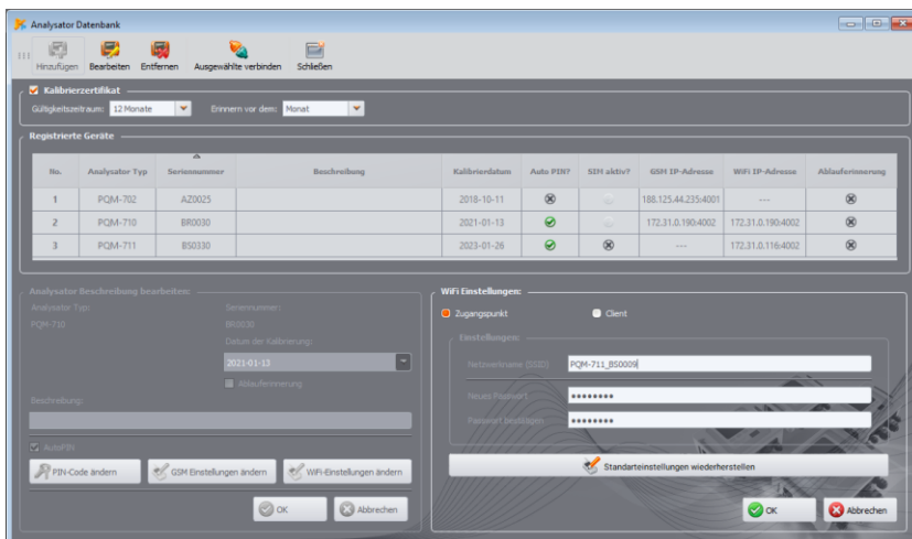
Abb. 42. Wi-Fi-Konfigurationsbildschirm im Online-Modus (Zugangspunktmodus auf dem Analysator).
