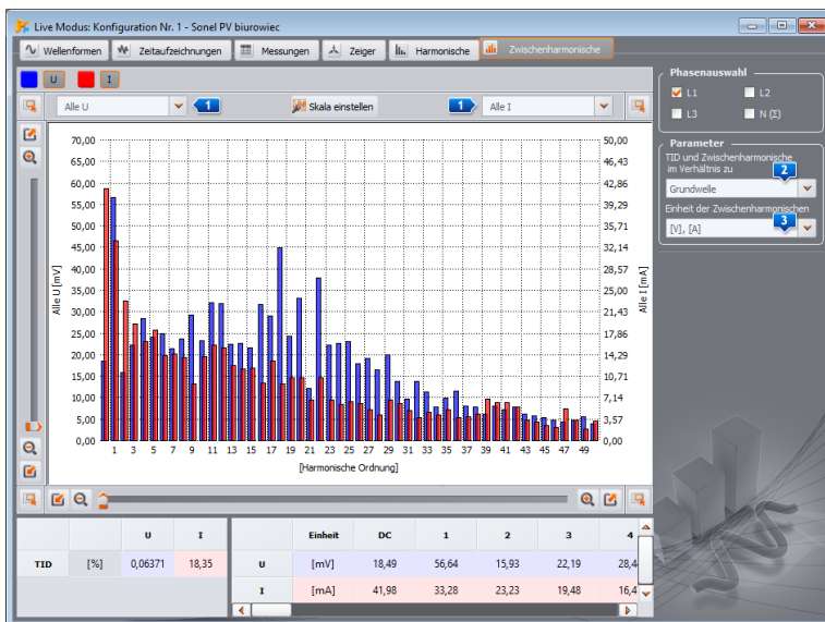
Abb. 52. Diagramm der Zwischenharmonischen
