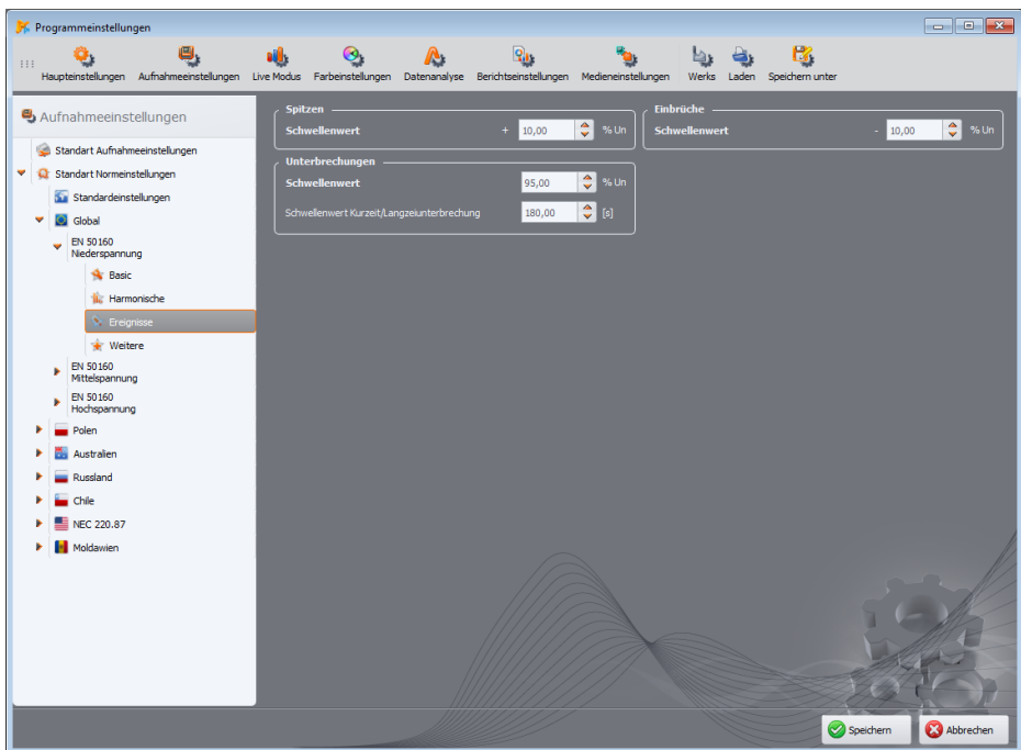
Abb. 80. Aufzeichnung nach EN 50160 - Ereigniseinstellungen.
