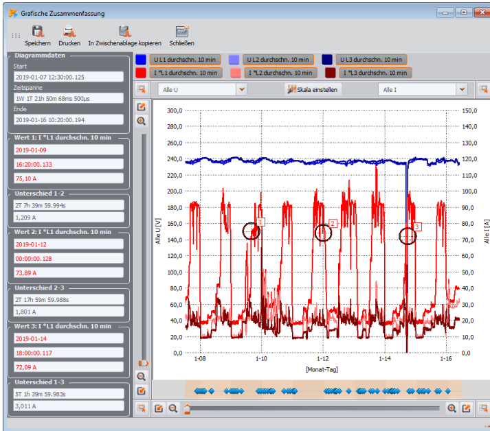
Abb. 68. Beispiel für eine grafische Zusammenfassung.
