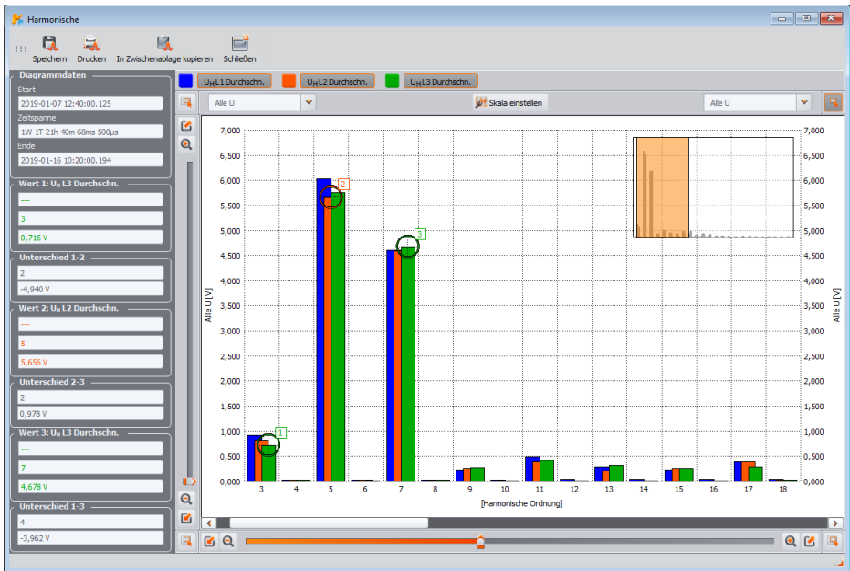
Abb. 61. Diagramm der Harmonischen
