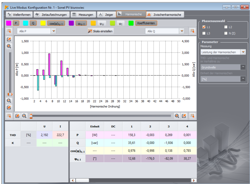
Abb. 51. Bildschirm für harmonische Leistung.
