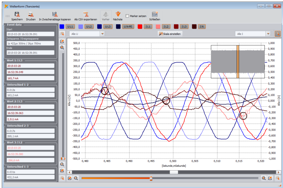
Abb. 72. Diagramm mit dem Anfangs- und Endoszillogramm des Ereignisses.
